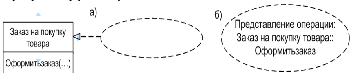
Рис. 3. Способы представления кооперации, которая реализует операцию класса
