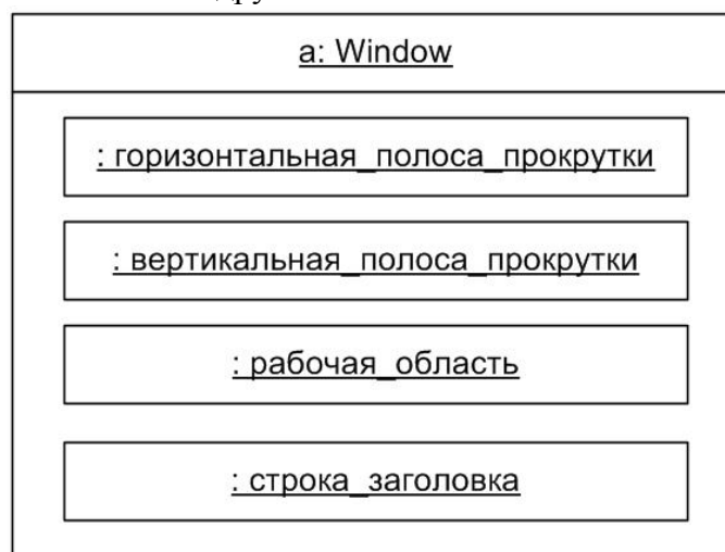
Рис. 8. Графическое изображение составного объекта на диаграмме кооперации
