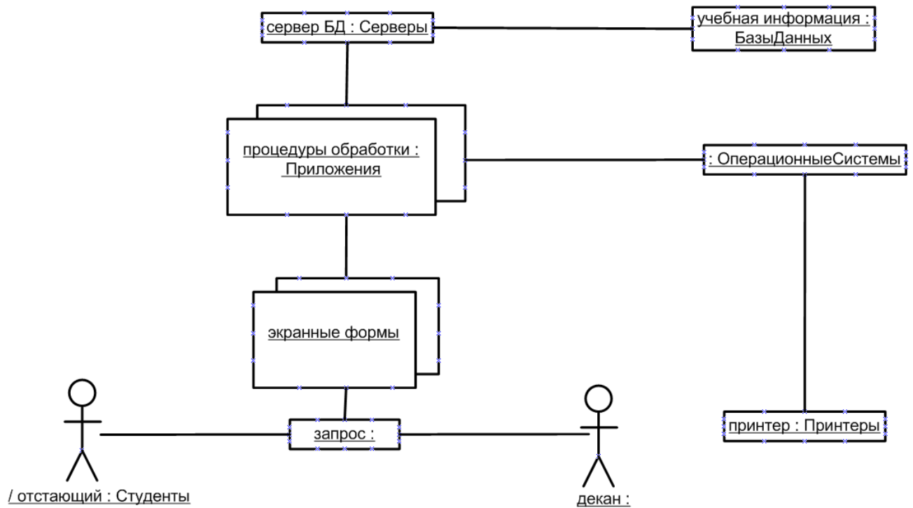
Рис. 11. Начальный фрагмент диаграммы кооперации для примера
