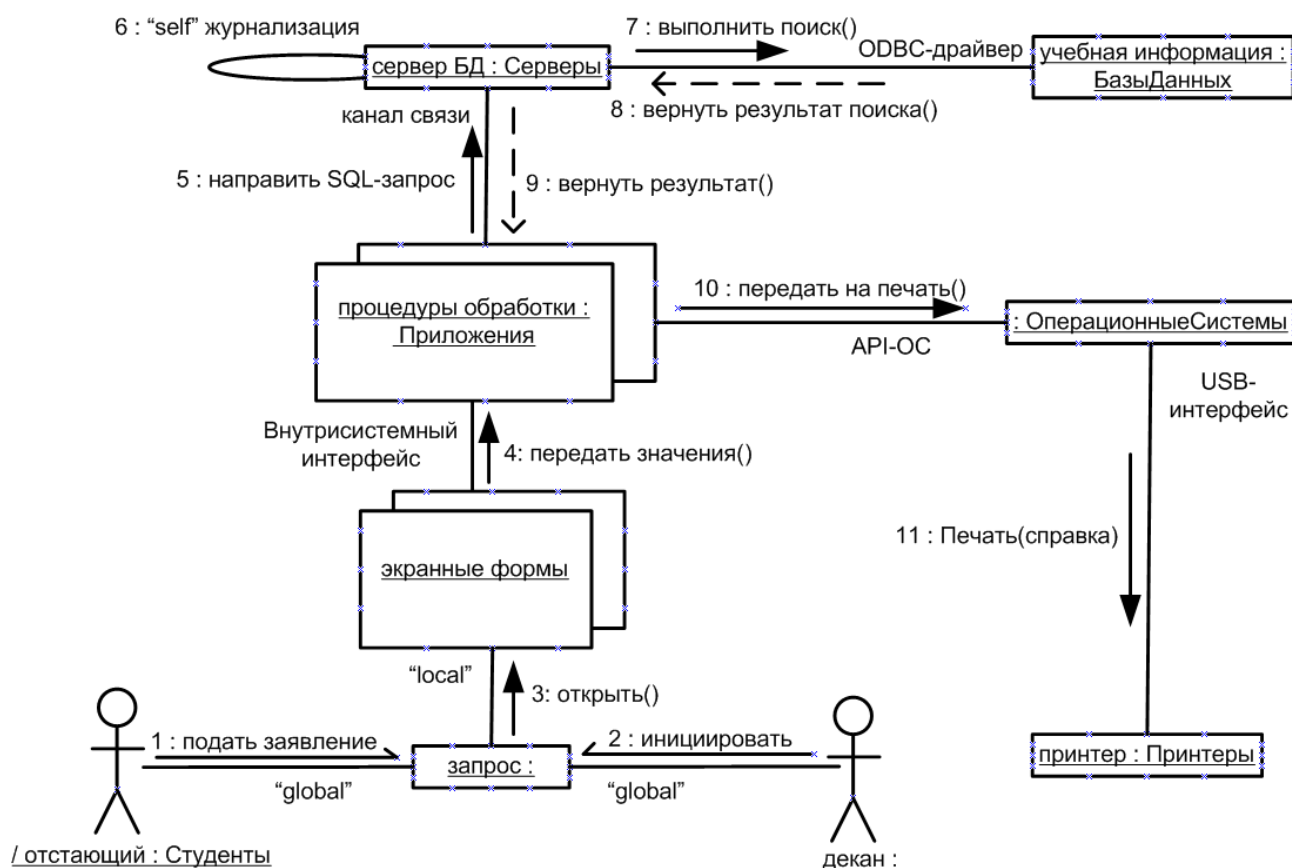
Рис. 13. Окончательный вариант диаграммы кооперации
