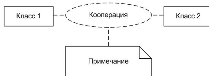
Рис. 1. Общее представление кооперации на диаграммах уровня спецификации
