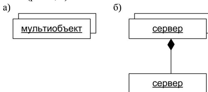
Рис. 5. Графическое изображение мультиобъектов на диаграмме кооперации
