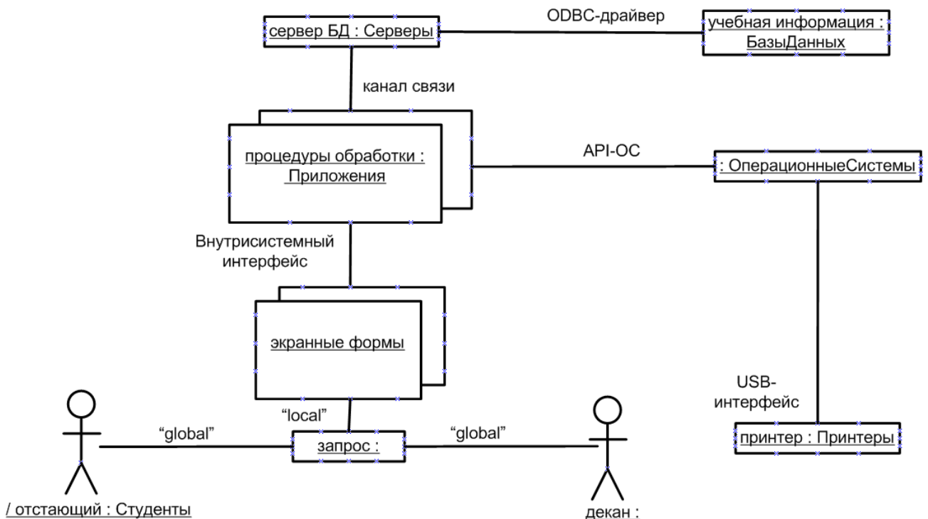
Рис. 12. фрагмент диаграммы кооперации, дополненный стереотипами ролей связей и именами ассоциаций
