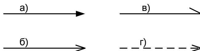
Рис. 10. Графическое изображение различных типов сообщений на диаграмме кооперации
